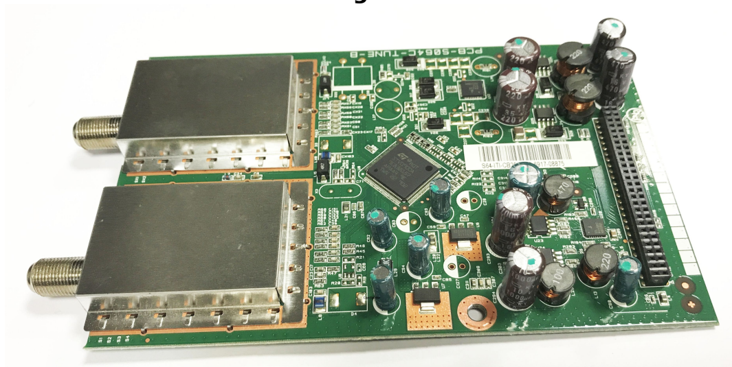
Podwójna głowica satelitarna DVB-S2 tunera nBox BZZB (ADB-5800SX) Enigma 2
