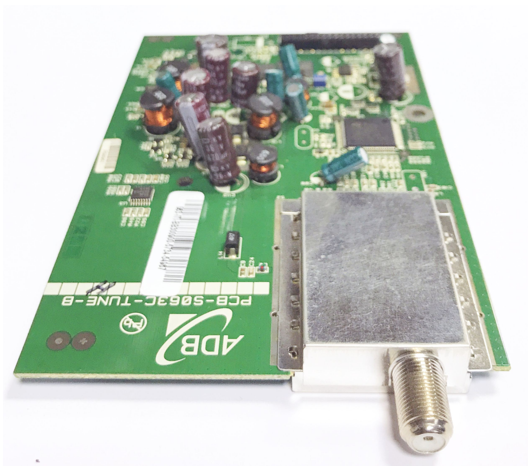
Podwójna głowica satelitarna DVB-S2 tunera nBox BZZB (ADB-5800SX) Enigma 2
